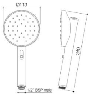
CAROMA RIVIERE VJET HANDSET
