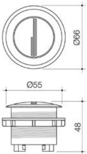
CAROMA BEZEL/BUTTON ROUND METAL
